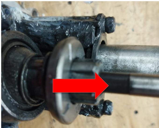
Obr.2 Poškodenie ozubeného prevodu
