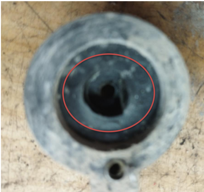
Obr.2 Poškodenie tiahla prepínača prevodových stupňov
