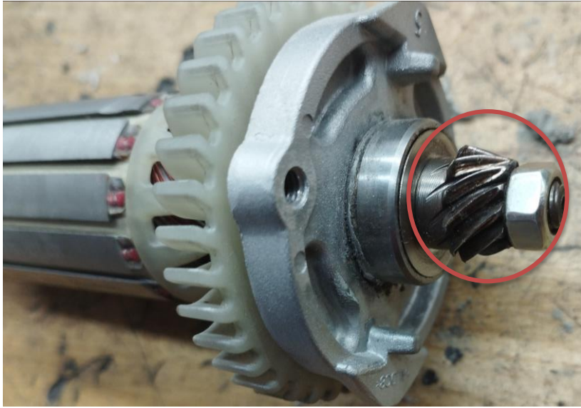
Obr.3 Opatrebnie primárneho ozubeného prevodu
